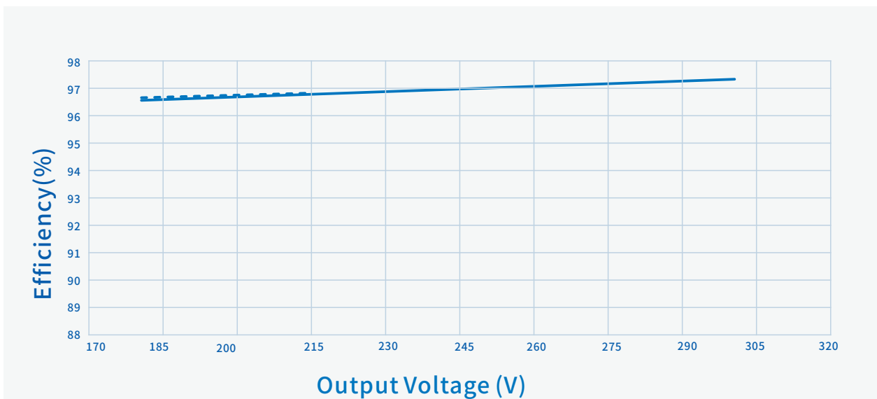
效率 Vs. 输出电压 (Vin=347Vac)
