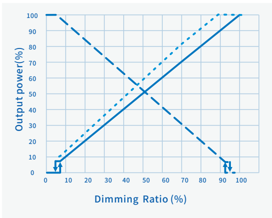
输出功率Vs.调光信号
