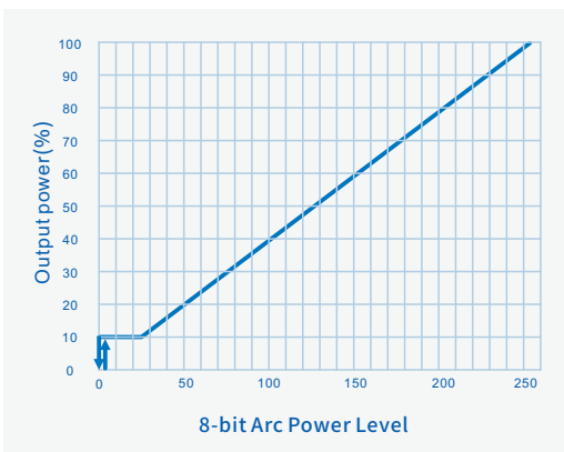
线性调光曲线
