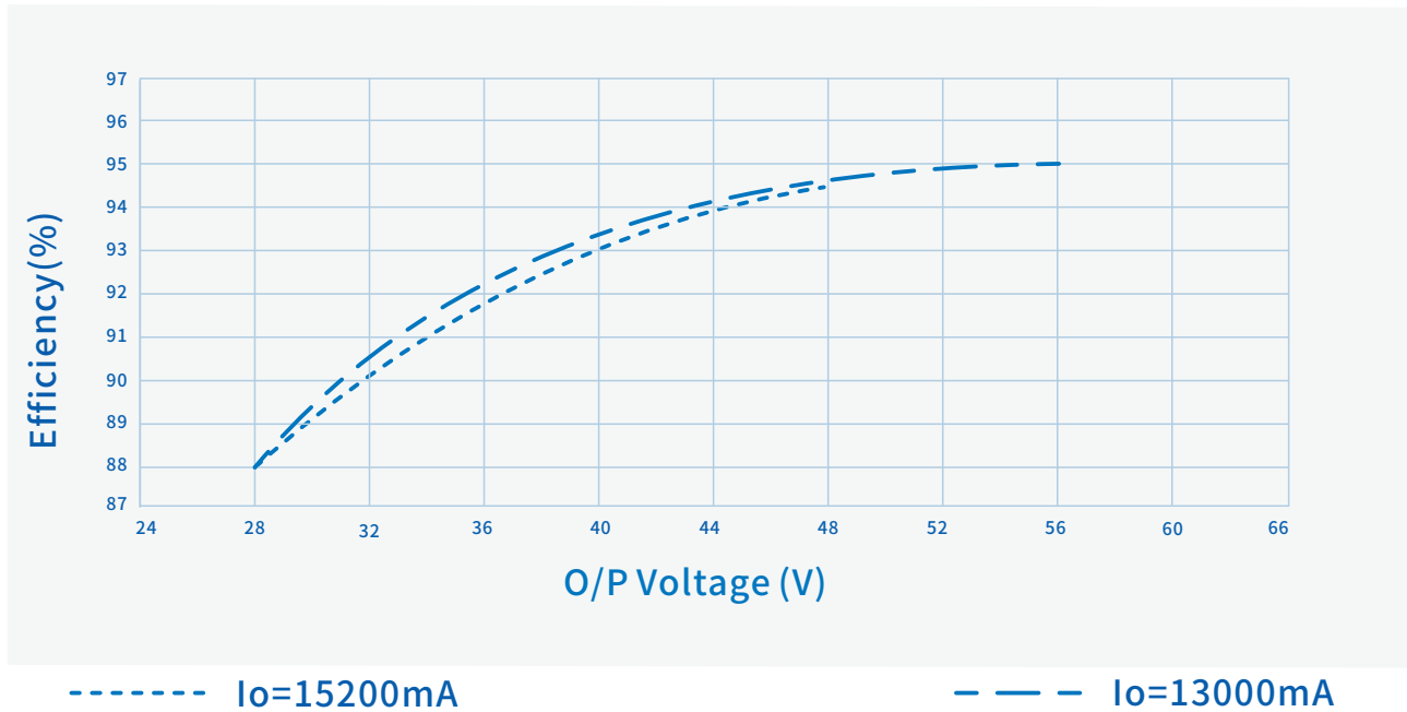
效率Vs. 输出( V_{in}=277V_{ac} )
