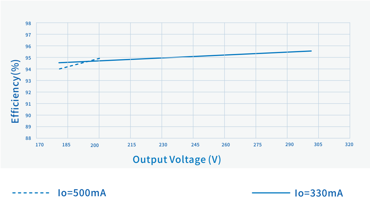
效率 Vs. 输出电压 (Vin=220Vac)
