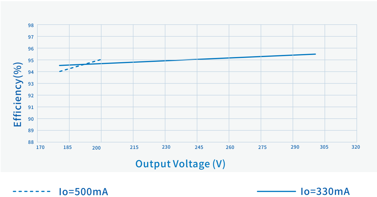
效率 Vs. 输出电压 (Vin=277Vac)
