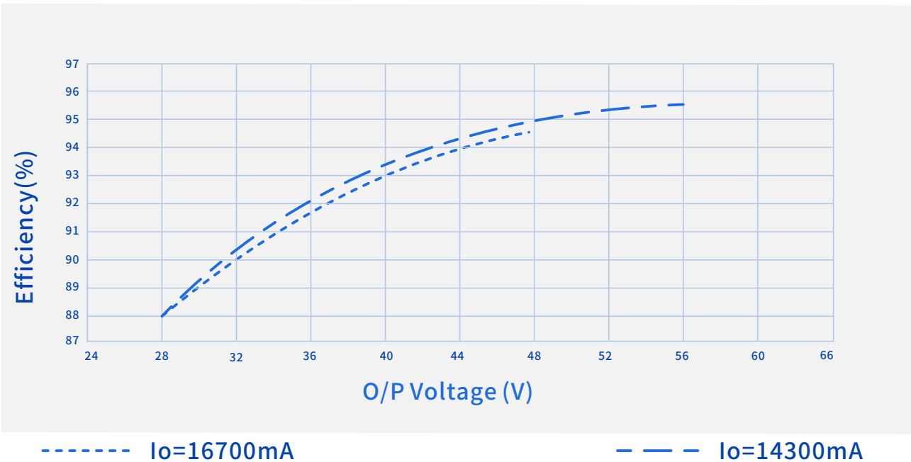
效率Vs. 输出(Vin=277Vac)
