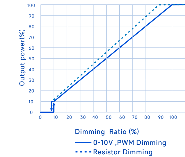
输出功率Vs.调光信号 (A/BHB机型)
