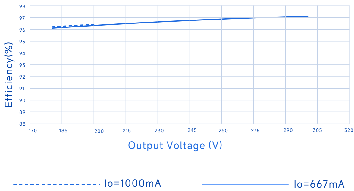
效率 Vs. 输出电压 (Vin=277Vac)
