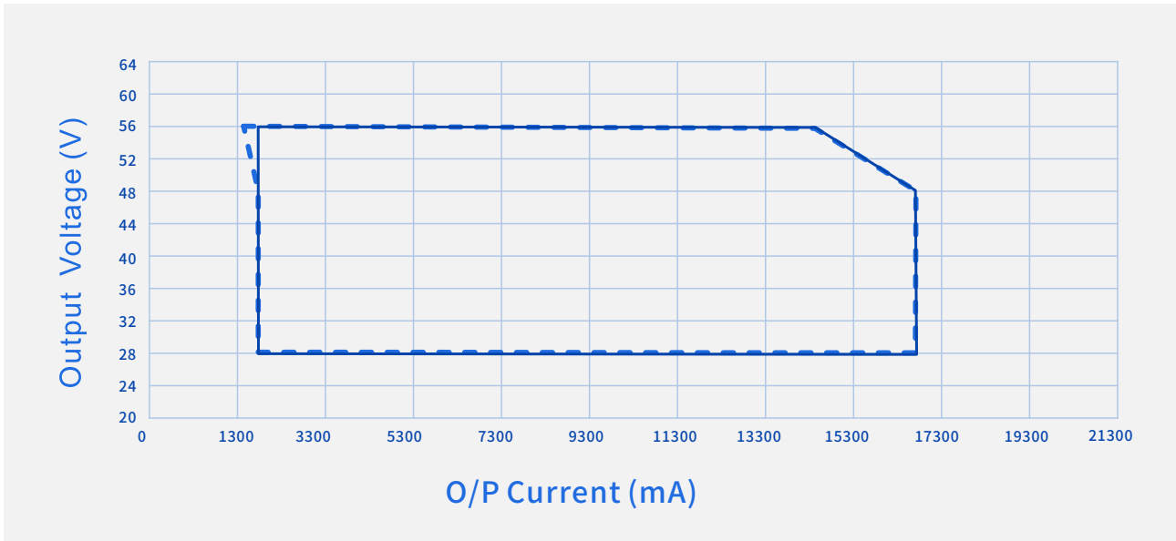
输出电压Vs.输出电流（调光/AOC窗口）
