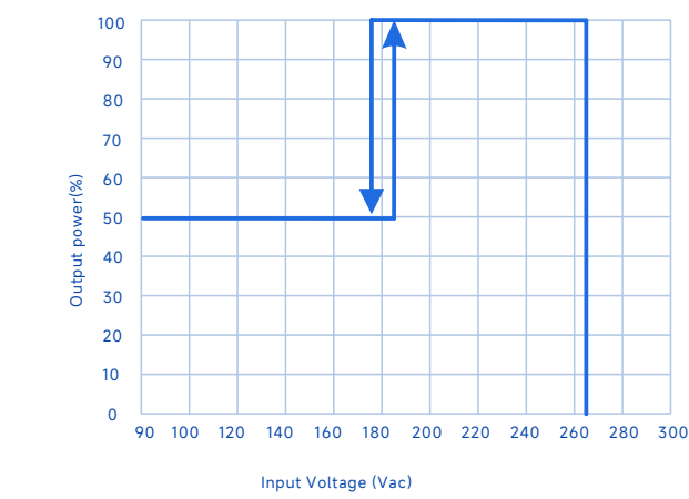
输入欠压降功率曲线
