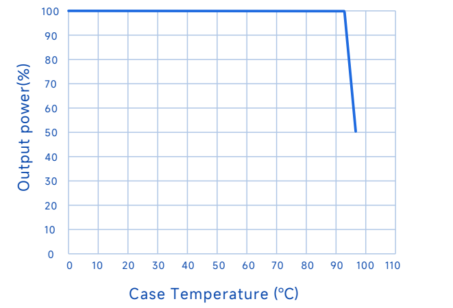
输出功率Vs.壳温
