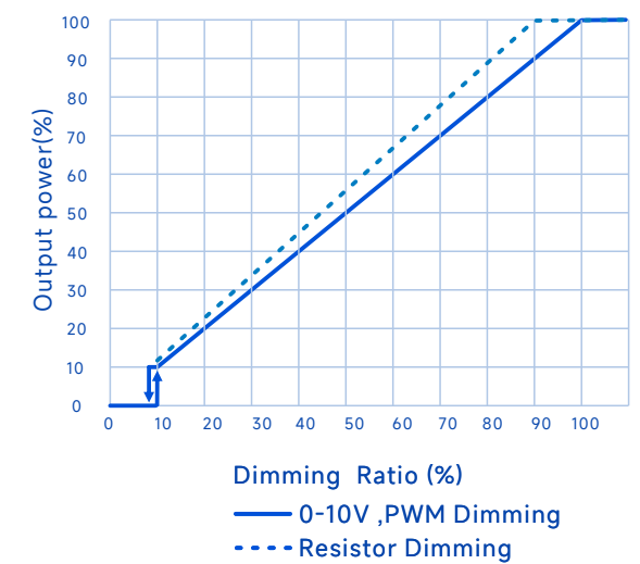
输出功率Vs.调光信号 (A/BHB机型)
