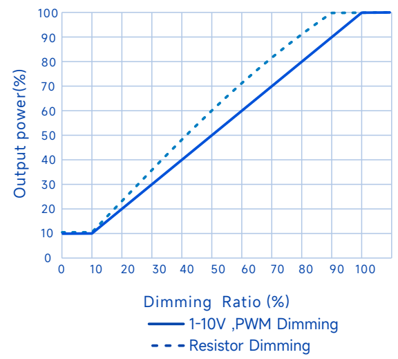
输出功率Vs.调光信号 (BB机型)
